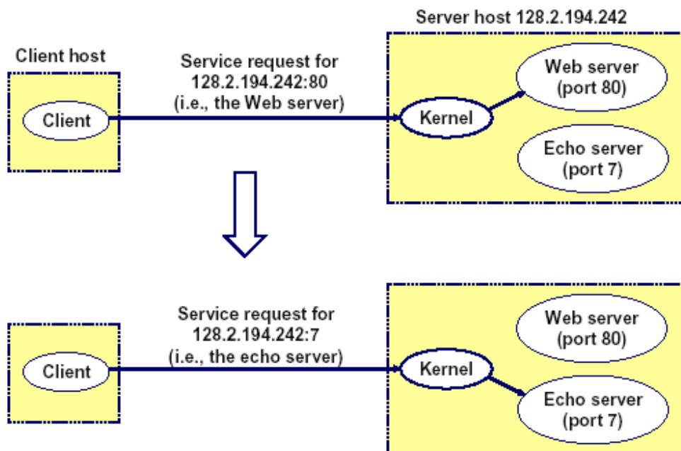
Gambar 9.3 Menggunakan Port untuk identifikasi service
