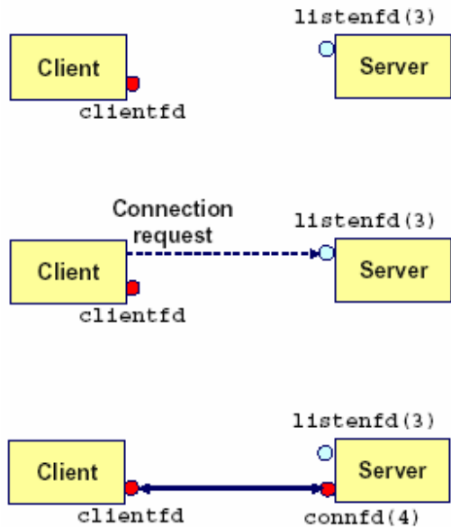
Gambar 9.5 Ilustrasi prosedur accept() antara client dan server
